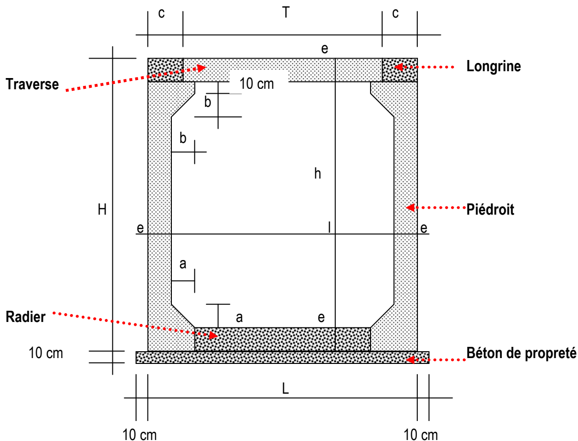
Plan de coffrage
