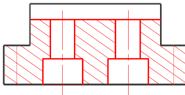
Coupe A-A
