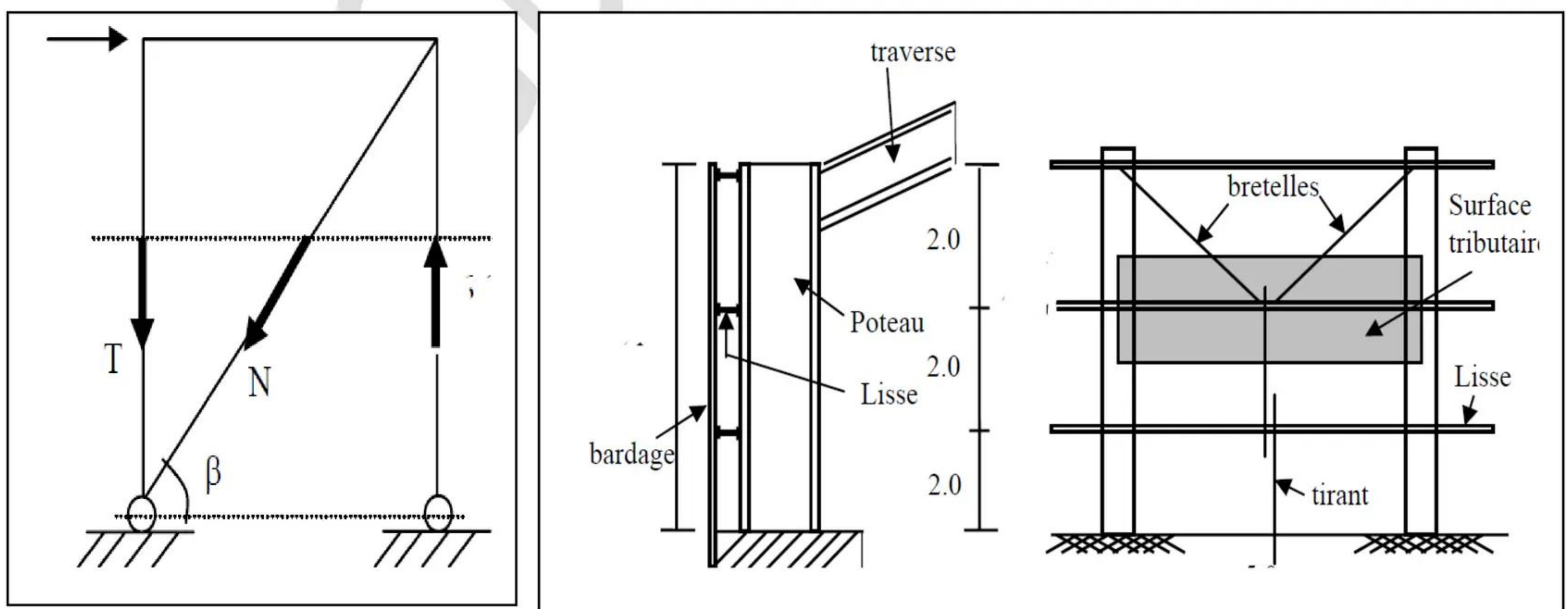
Figure 3.2. Éléments tendus dans une ferme (diagonales, liernes)
