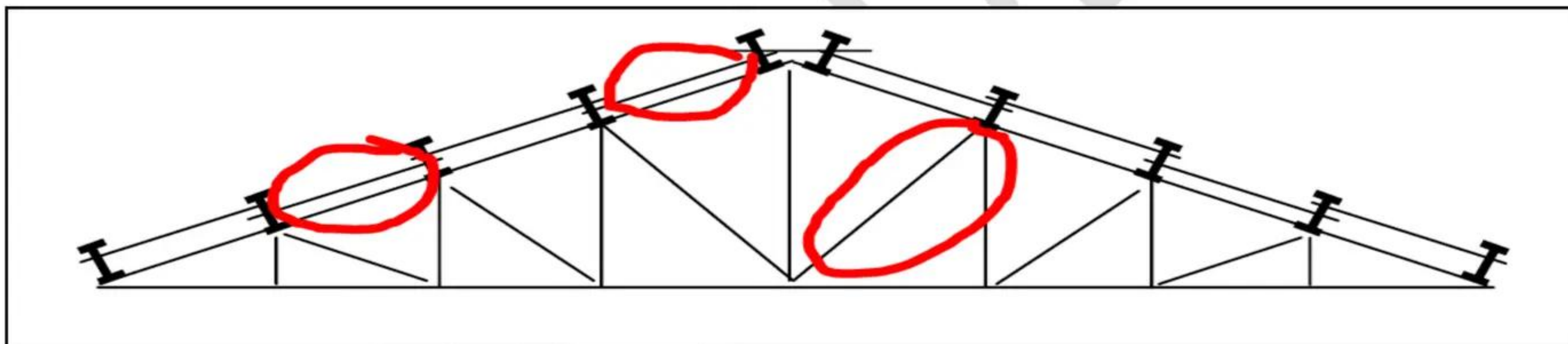
Figure 3.2. Éléments tendus dans une ferme (diagonales, liernes)
