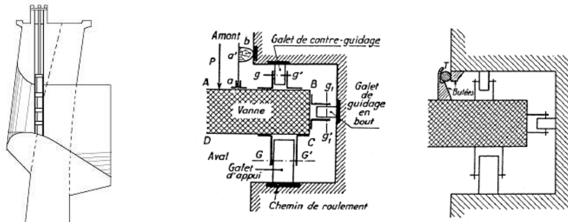
Figure 59 : Coupes types d'une vanne wagon (Delliou, 2003)
