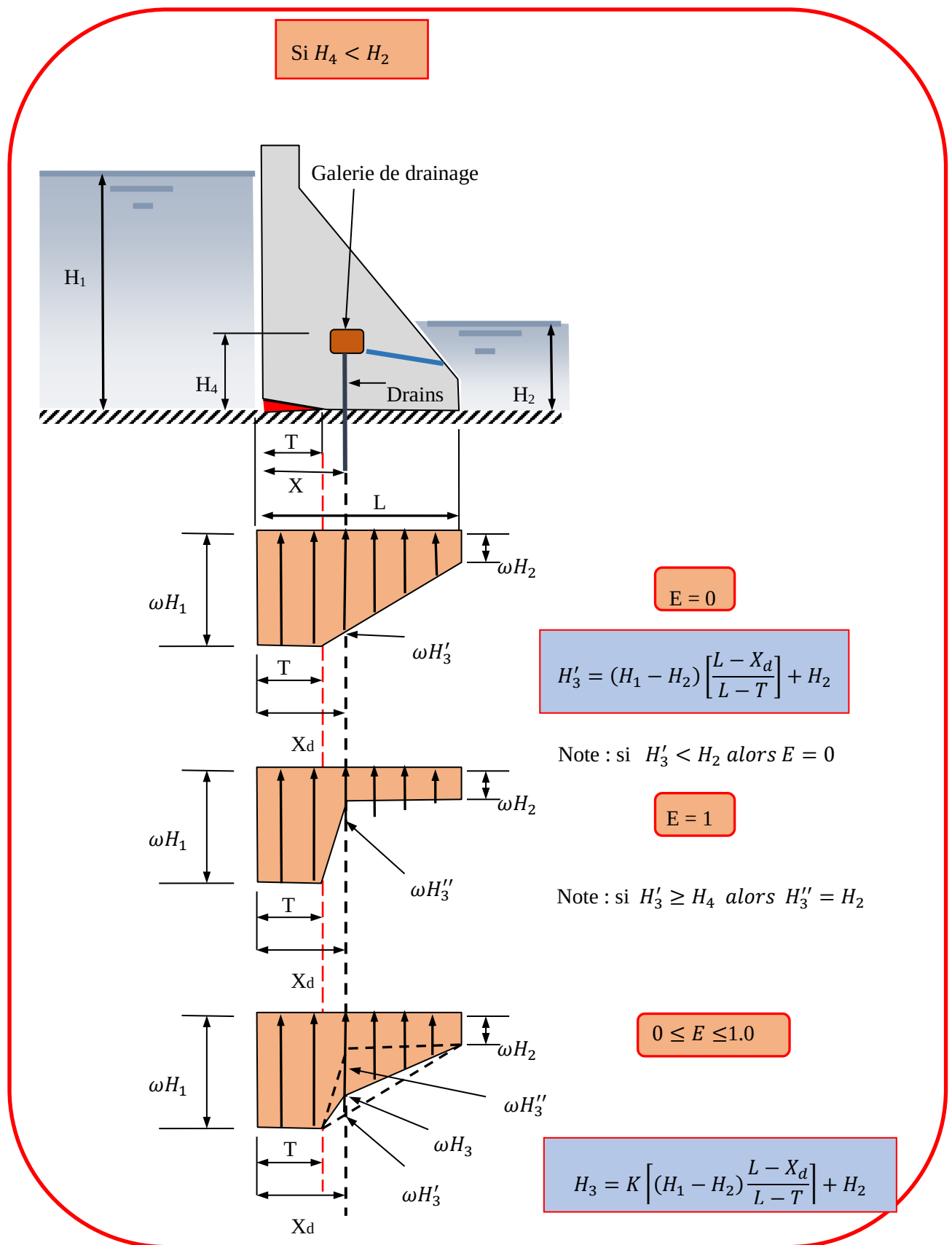
Figure 20 : La répartition des sous-pressions en présence d'une fissure Si H_4 < H_2 (Schleiss and Pougatsch, 2011)
