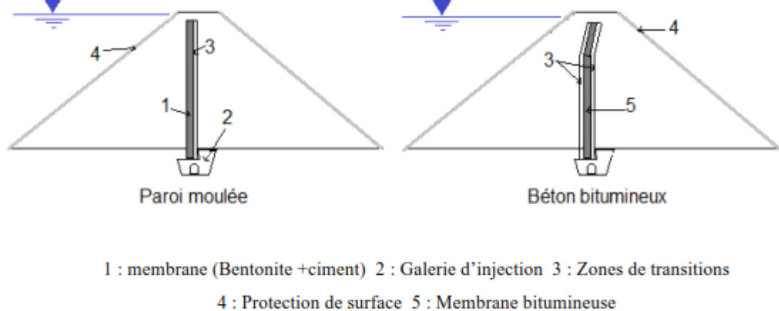
Figure 39 : Barrages en remblai avec membranes centrales (Lehbab, 2019).
