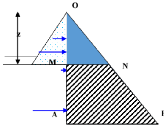
Figure 25 : Schéma simplifié pour le calcul de la stabilité au renversement
