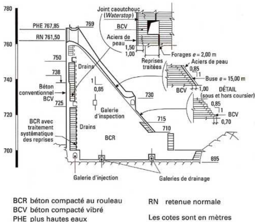
Figure 11 : Barrage poids BCR (Carrère, 1996)
