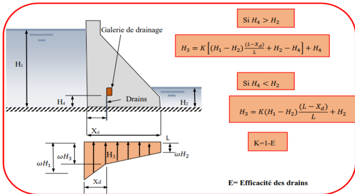
Figure 17 : Sans fissuration le cas où la hauteur du drain supérieure à la hauteur d'eau aval ( H_4 > H_2 ) (Schleiss and Pougatsch, 2011)
