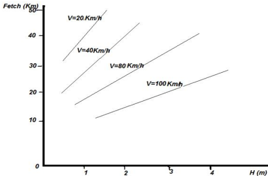
Figure 46 : Variation de la hauteur des vagues en fonction du Fetch et du vent
