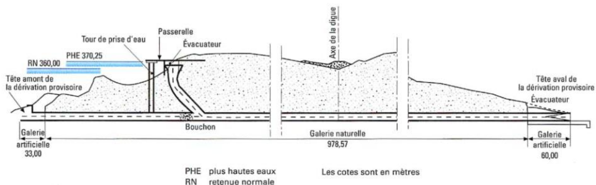
Figure 55 : Évacuateur à puits et tunnel (Hammam Debagh, Algérie) (Carrère, 1996).
