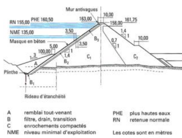
Figure 53 : Barrage à masque en béton de Khao Laem (Thaïlande) (Carrère, 1996)
